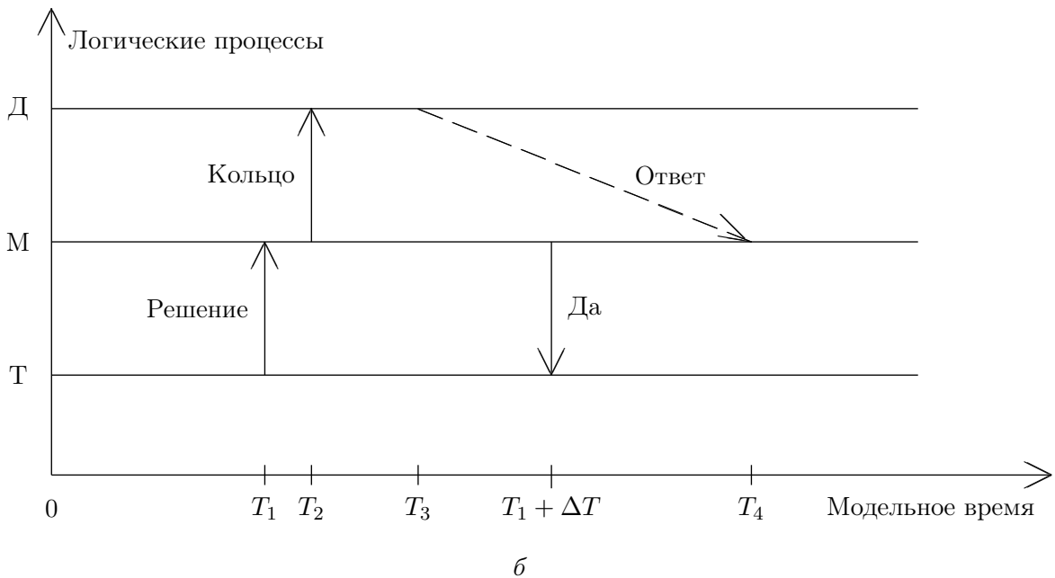
Рис. 3. Временная диаграмма исполнения модели: а — корректная имитация; б — некорректная имитация.
